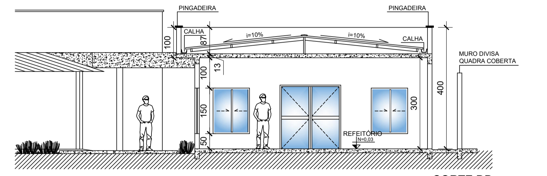
CORTE DD ESC. 1:75
