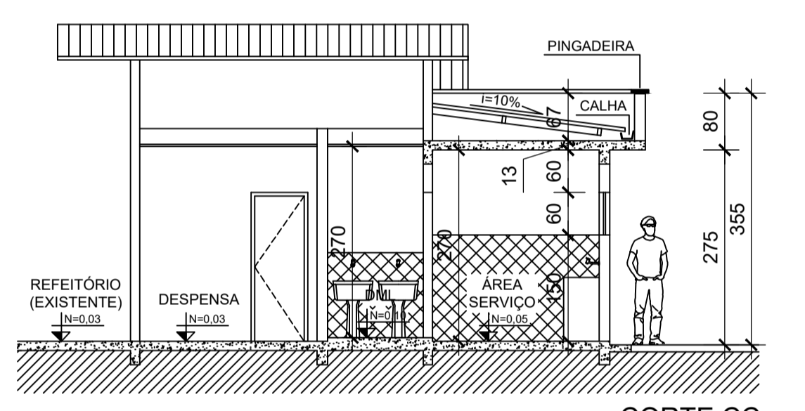
CORTE CC ESC. 1:75
