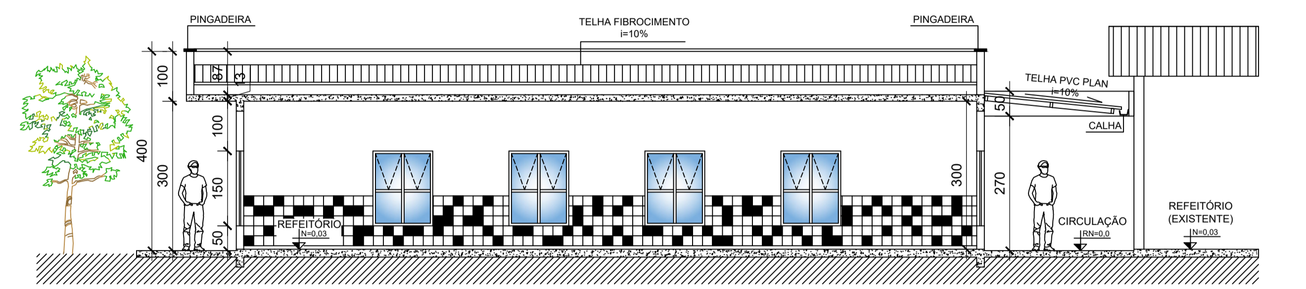
CORTE BB ESC. 1:75
