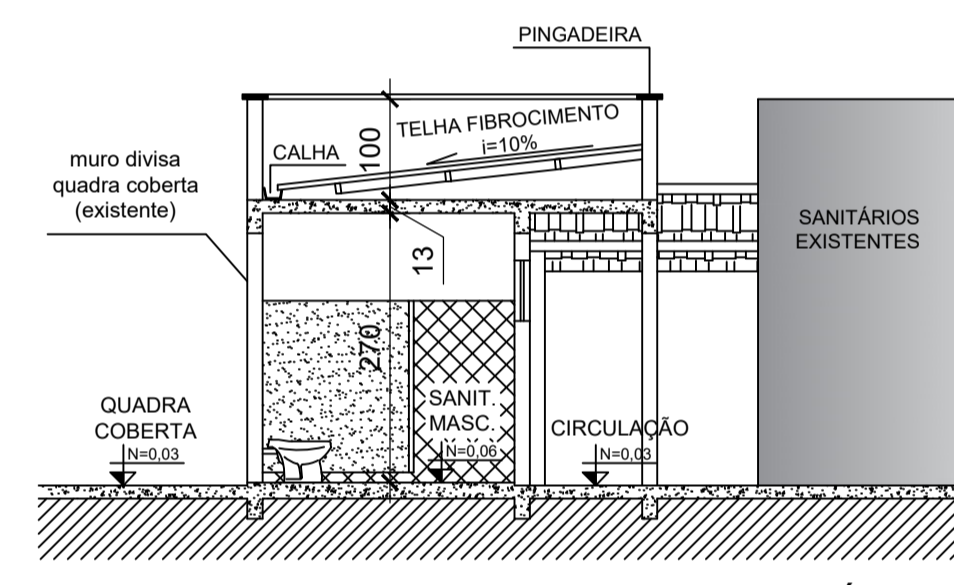
CORTE SANITÁRIOS ESC. 1:75
