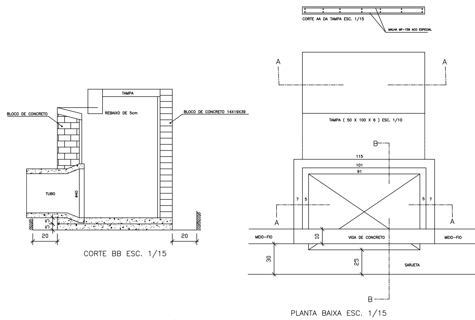
DETALHE - BOCA DE LOBO
